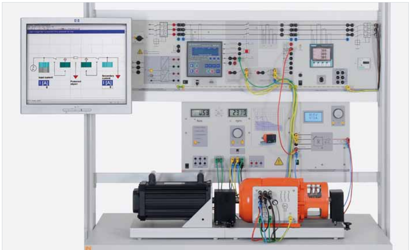
Versuchsbeispiel „Generatorschutz EGP 1“
